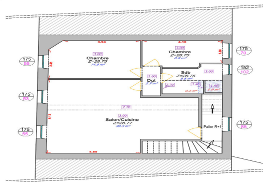
1er ETAGE
